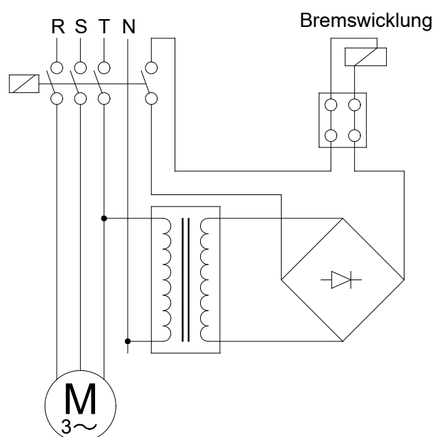
Schnelle Bremsung (24 V)
