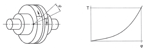
Rigidité du ressort à barre de torsion et angle de torsion
