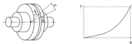
Rigidità elastico torsionale e angolo di torsione
